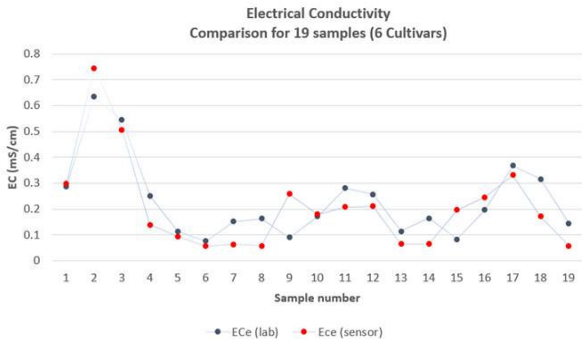
Abbildung 13: EC-Werte aus einem Praxisbetrieb im Vergleich – die trendmäßige Korrelation ist deutlich erkennbar.
