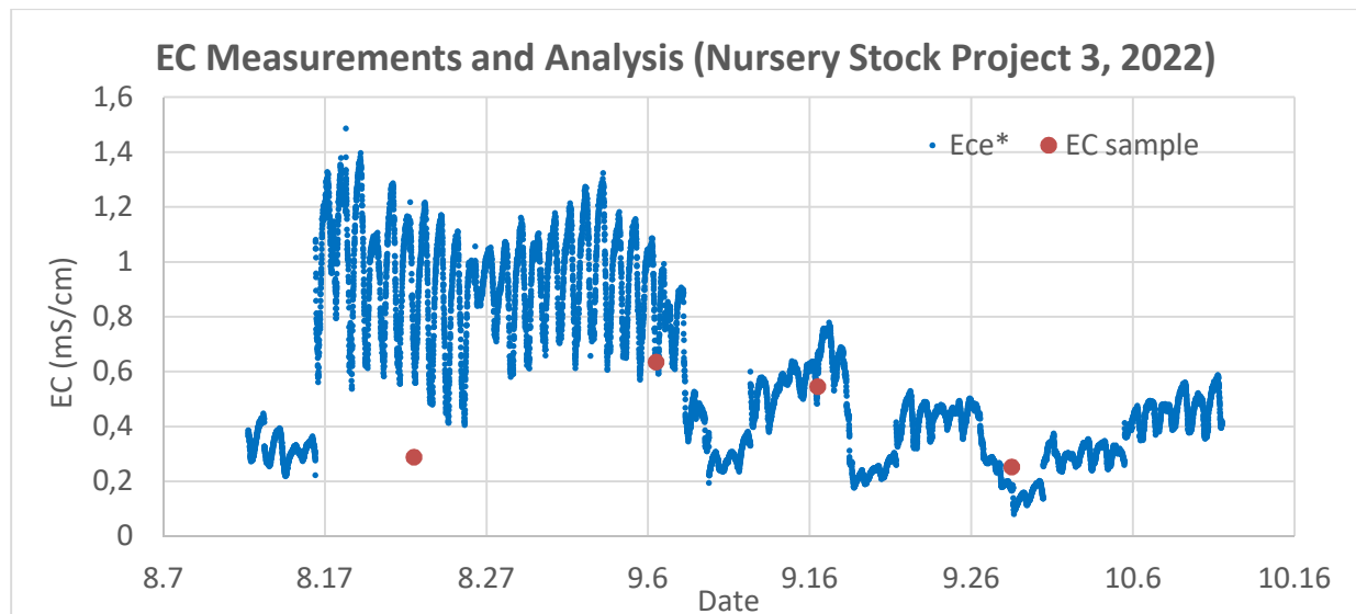
Abbildung 14: EC-Werte aus einem Praxisbetrieb „in realtime“ vor der Begradigung: Die Häufigkeit der Messintervalle erschwert das Ablesen und die Interpretation der Werte.
