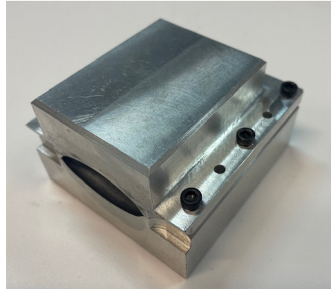
Abbildung 6: Prototyp einer Aluminiumgussform zum Gießen der Leiterplatte
