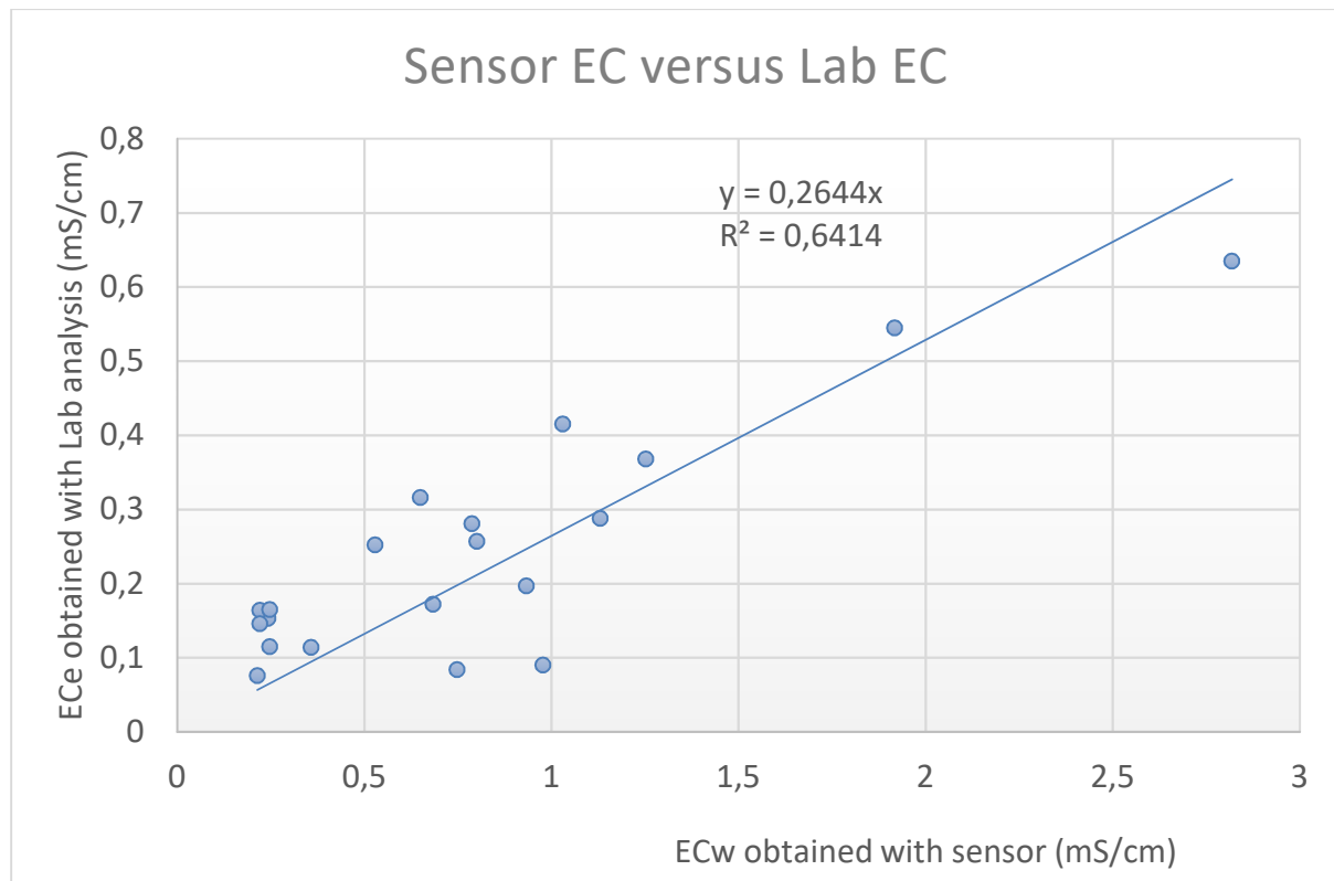
Abbildung 12: EC-Werte, gemessen mit dem Sensor und im Labor im Vergleich
